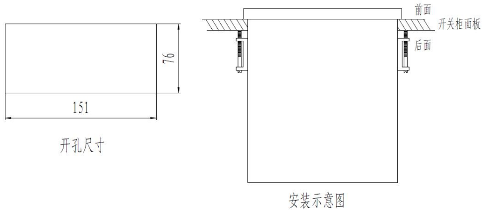
图 4（安装尺寸）
