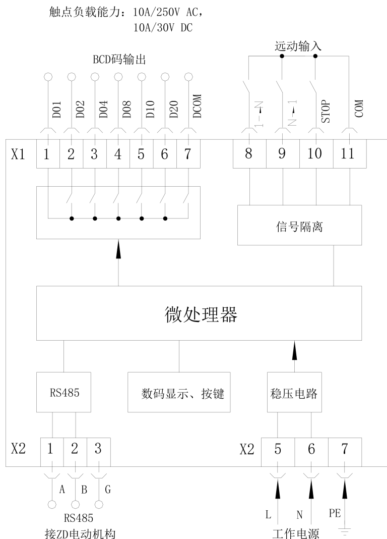
图 5（电路方框图）
