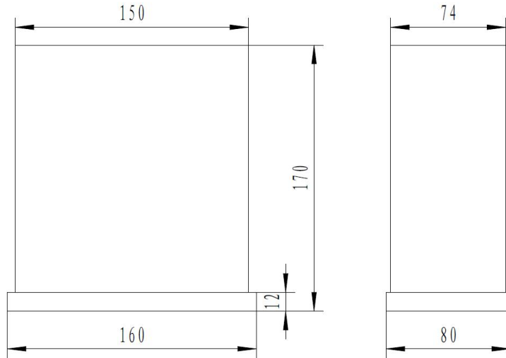
图 3（外形尺寸）
